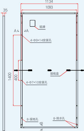
后视图
