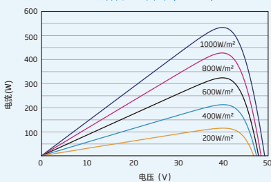
组件的P-V曲线 (535W)
