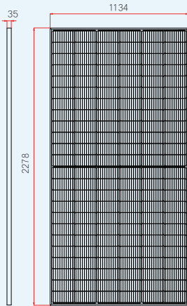
正视图
